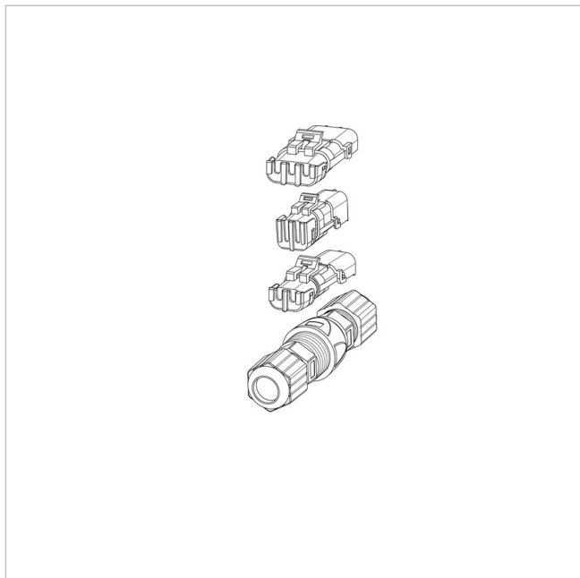
Anschlusskit für Bosch MIC7000, IP67, 5 Stück
