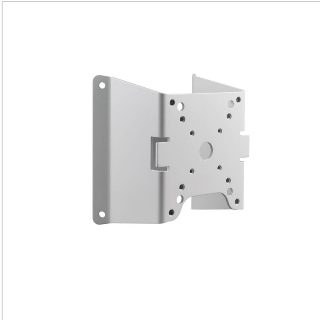
Adapterplatte für Eckmontage für Bosch Kameras
