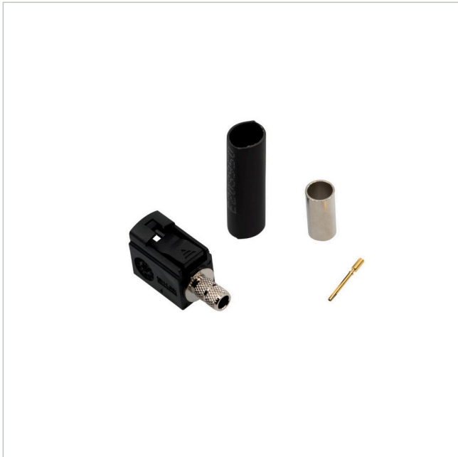
Crimpset mit FAKRA- Steckverbinder, 10er-Pack
