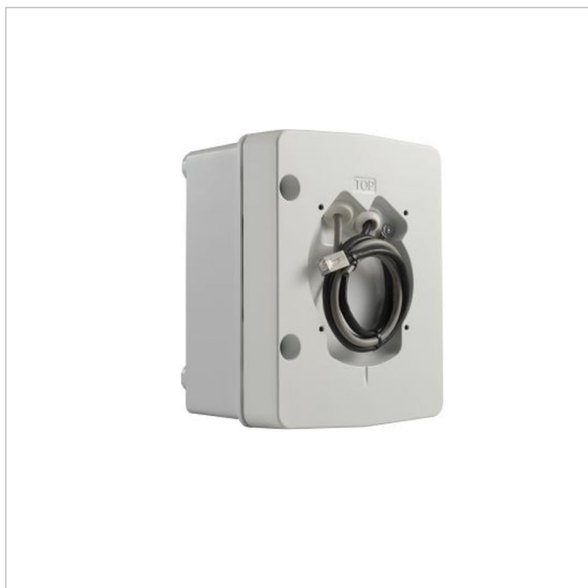
Anschlussbox für Bullet 148mm ohne Netzteil, IP66
